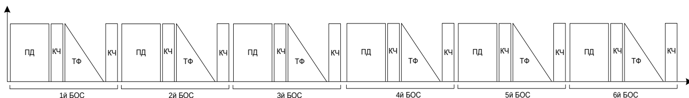
Рисунок 19 – Возможные варианты распределения спектра в полосе 48 кГц
