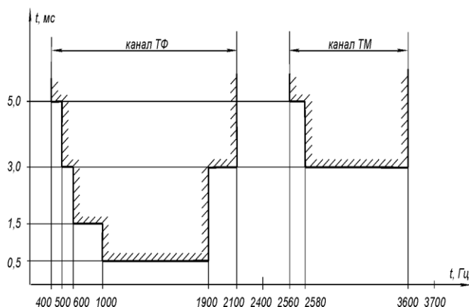
Рисунок 8 – Отклонение группового времени прохождения комбинированного канала ТЧ (ТФ+ТМ) с полосами от 0,3 до 2,4 и от 2,56 до 3,7 кГц
