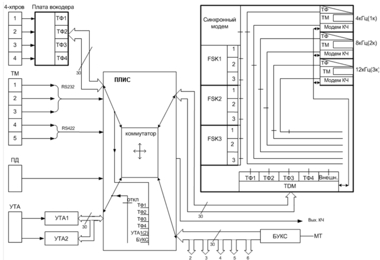
Рисунок 14 – Структурная схема БОС
