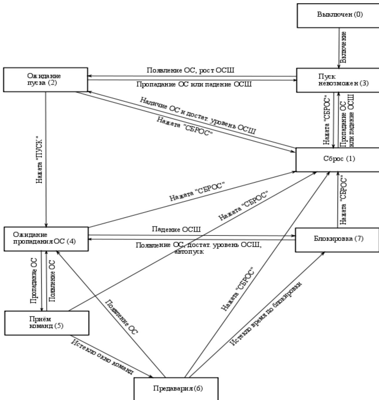
Рисунок 26 — Возможные переходы состояний приёмника блока РЗПА
