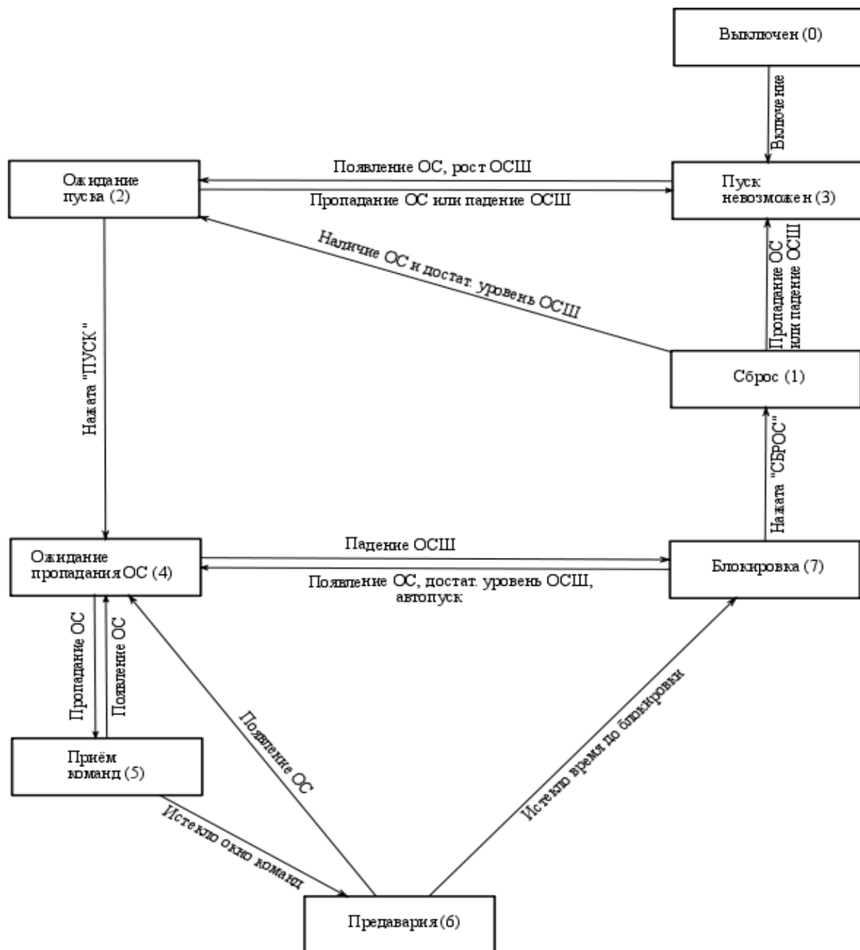
Рисунок 25 — Типичные переходы состояния приёмника блока РЗПА
